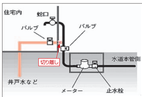
図 クロス配管の例
