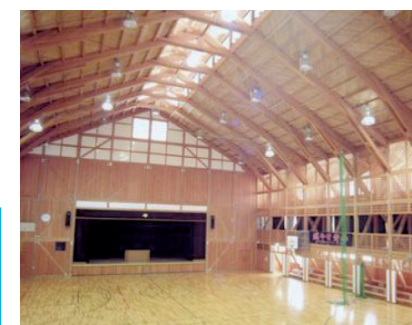
全国的にも珍しい木造の加美中体育館
